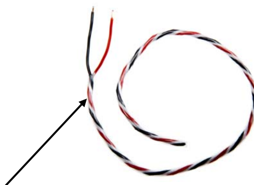
højttalerens indvendige kabelføring er udført med det amerikanske Nordost Spellbinder kabel
